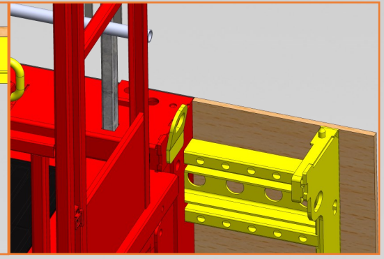
Contreplaqué epr=18mm affleurant avec tôle coffrante inox et filant pour côte bloquée
