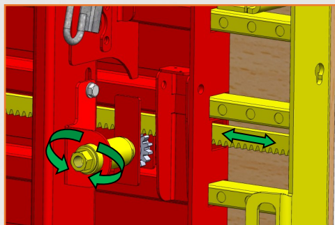
Déplacement extension par crémaillère
