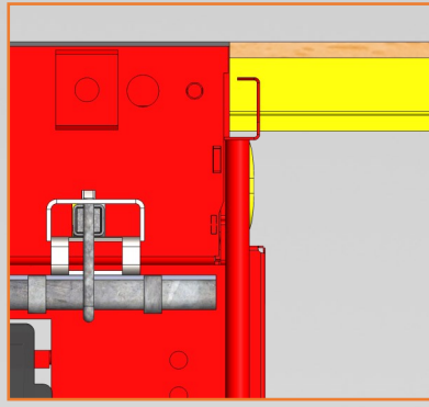
Contreplaqué epr=18mm affleurant avec tôle coffrante inox et filant pour côte bloquée
