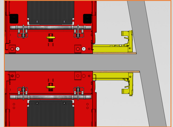
Utilisation en reprise de voile inclinée
