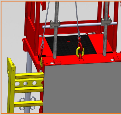
Levage vertical en 2 points.
