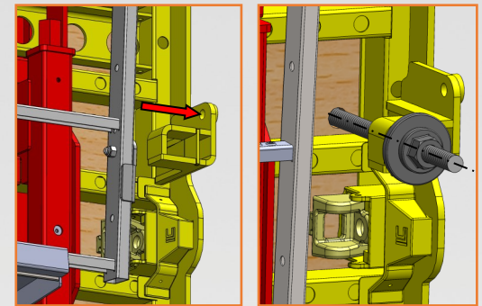
Support pour clamage et support pour entretoise
