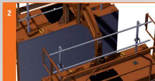
Protection côté face coffrante escamotable sans chaînes.
