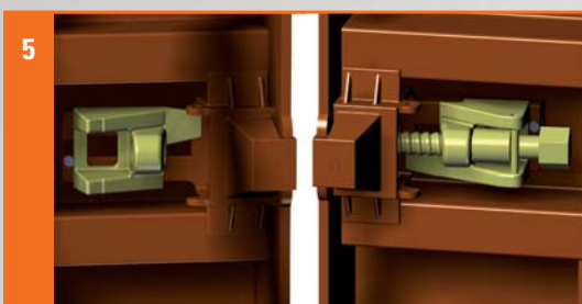
Verrous de BAAM mâle et femelle imperdables. Nouveaux modèles brevetés.
